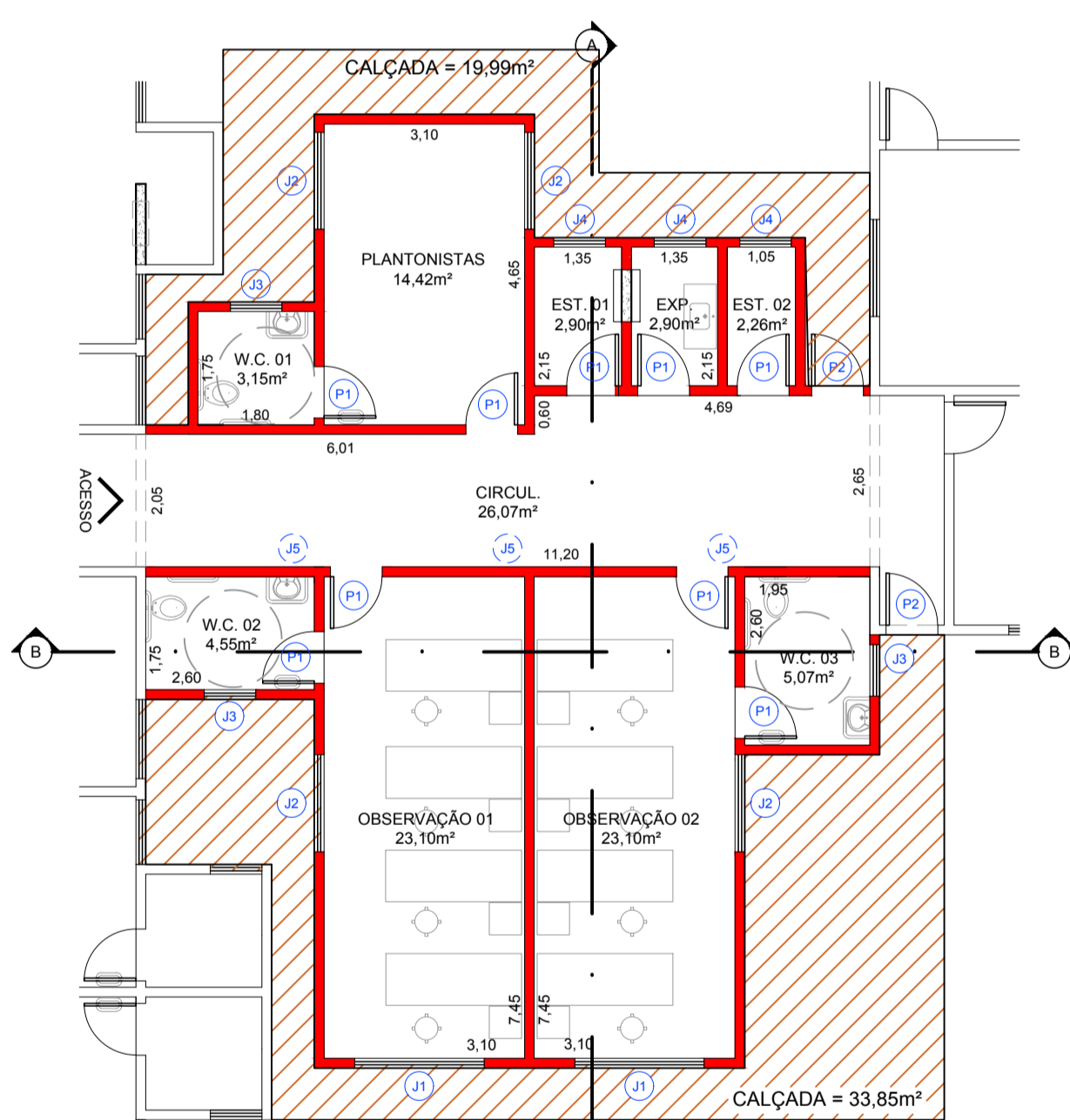
PLANTA ESCALA 1/100
