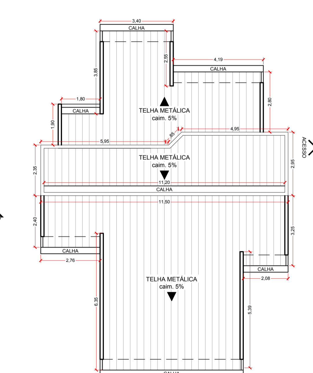
COBERTURA ESCALA 1/100
