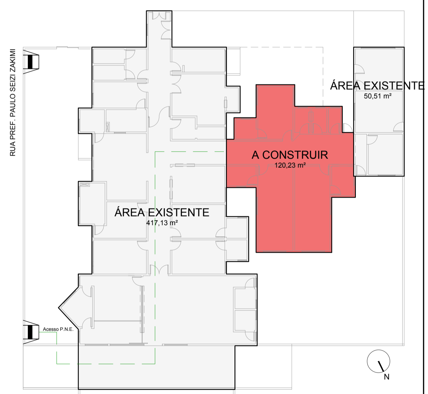
IMPLANTAÇÃO ESCALA 1/200
