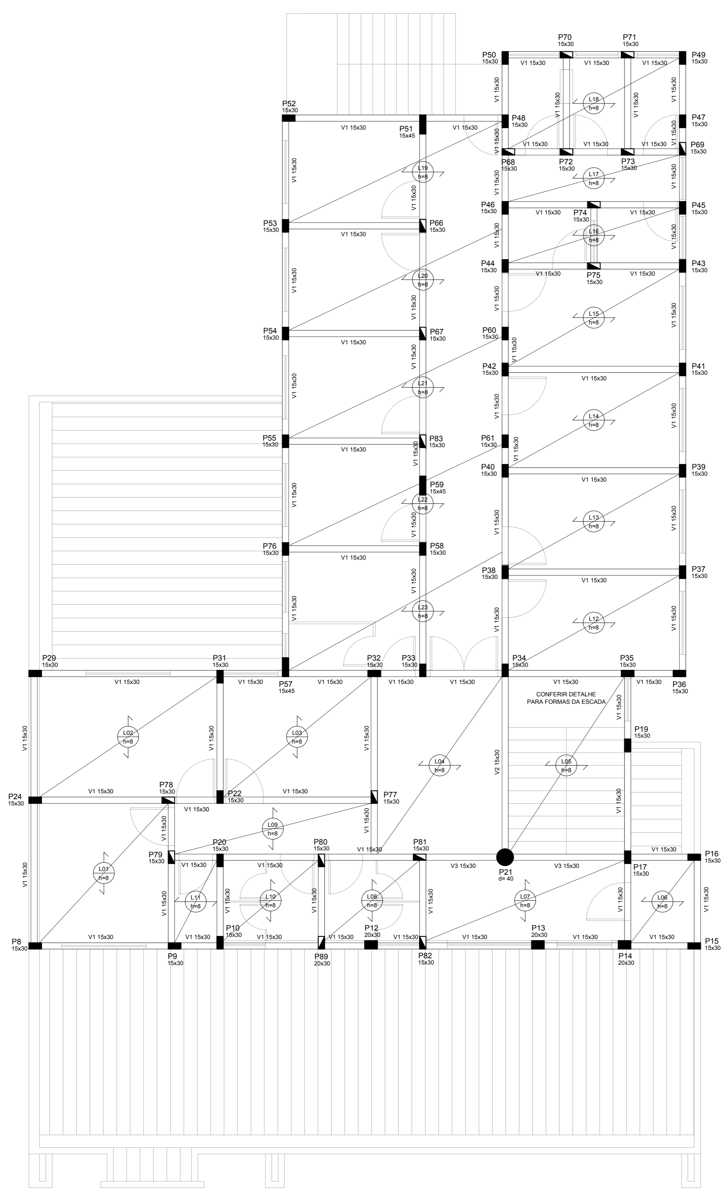
FORMA DO SUPERIOR - PILARES, VIGAS E LAJES ESCALA 1:50
