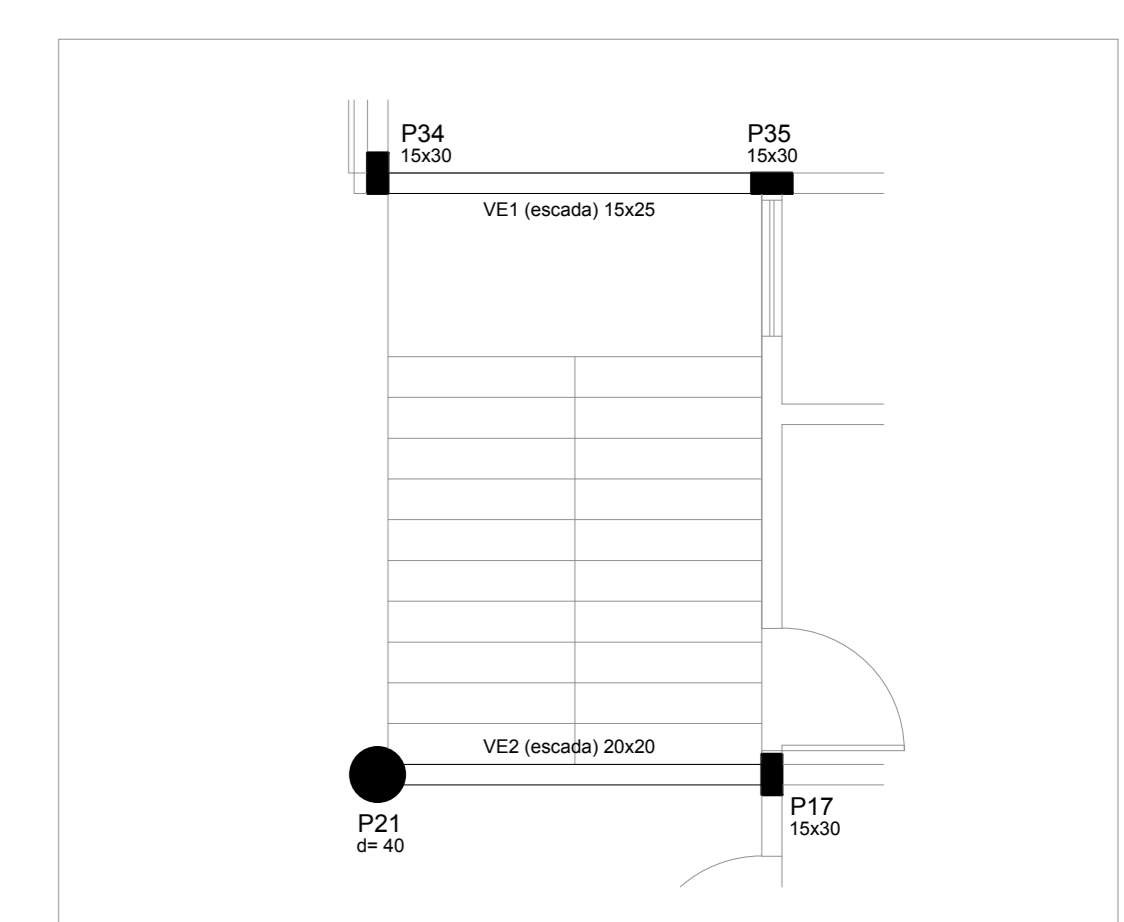
FORMA DOS PILARES E VIGAS ESCADA INTERNA ESCALA 1:50
