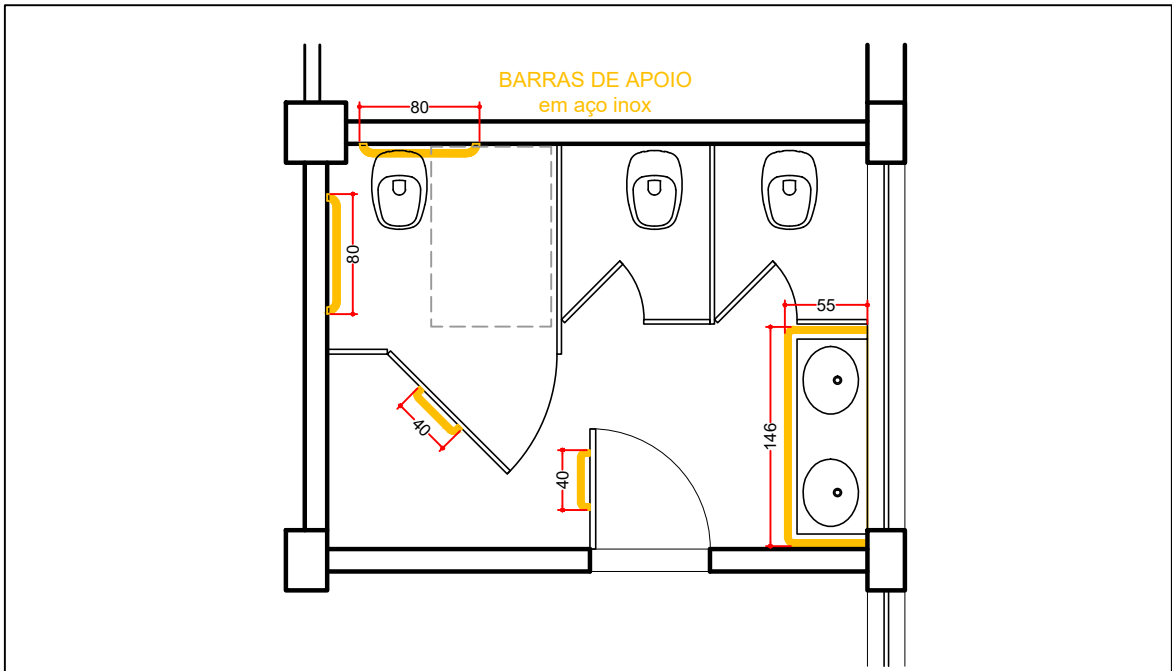
SANITÁRIO TIPO - FUNCIONÁRIOS (02 NO PAV. TÉRREO E 02 NO PAV. SUPERIOR) ESCALA 1:50
