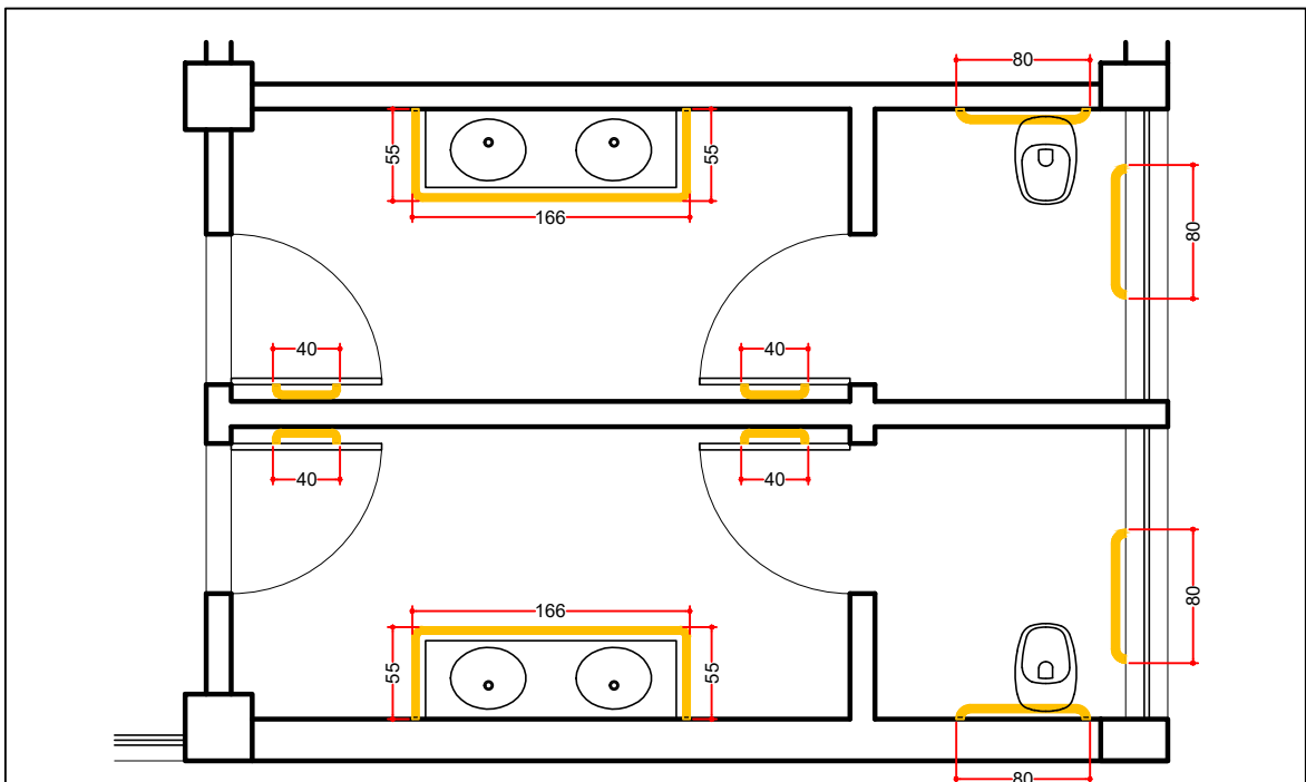
SANITÁRIOS P/ PÚBLICO (PAVIMENTO TÉRREO) ESCALA 1:50
