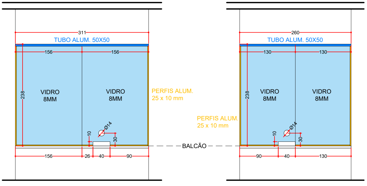
TELEFONISTA / PROTOCOLO ESCALA 1:50
