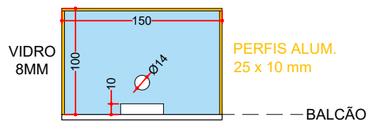
BALCÃO (09 UNIDADES) ESCALA 1:50
