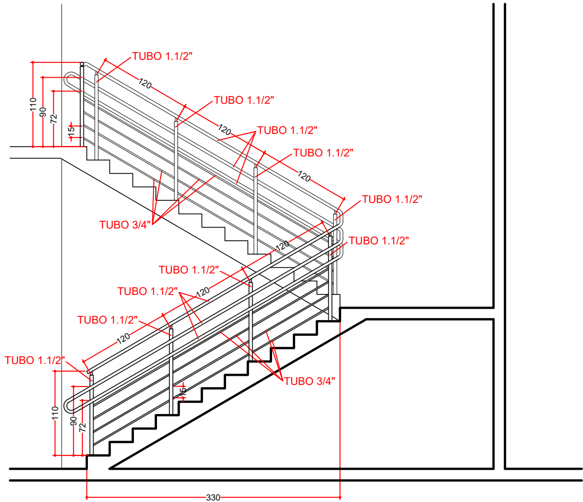
ESCADA INTERNA FUNCIONÁRIOS ESCALA 1:50
