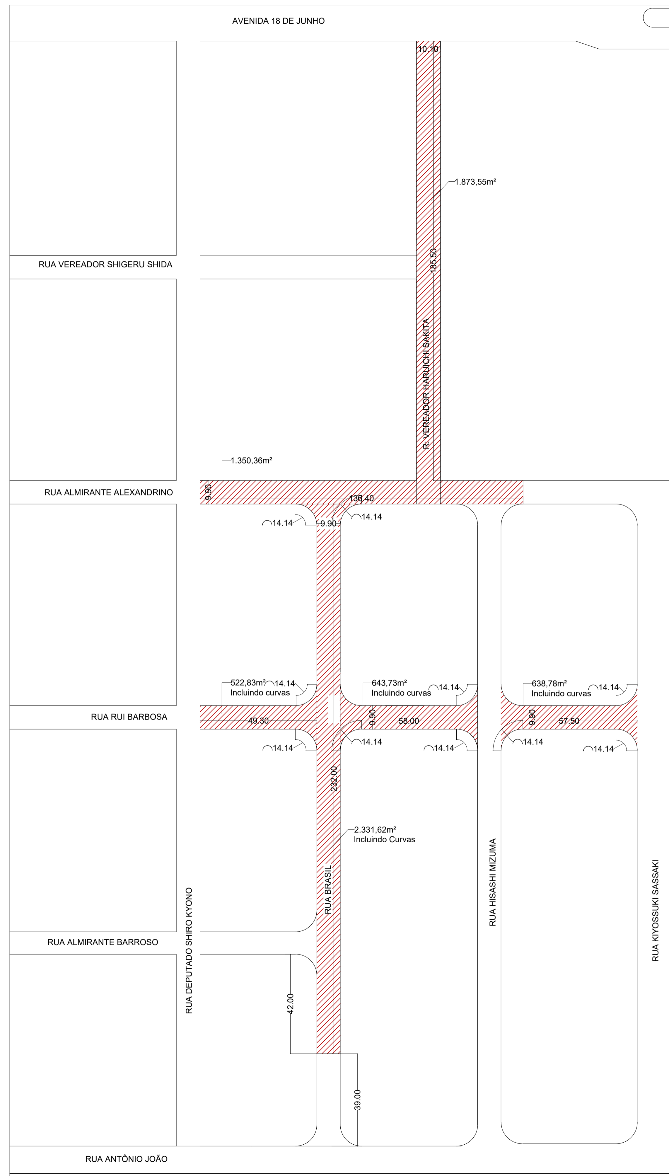
PLANTA ESC: 1/1000
