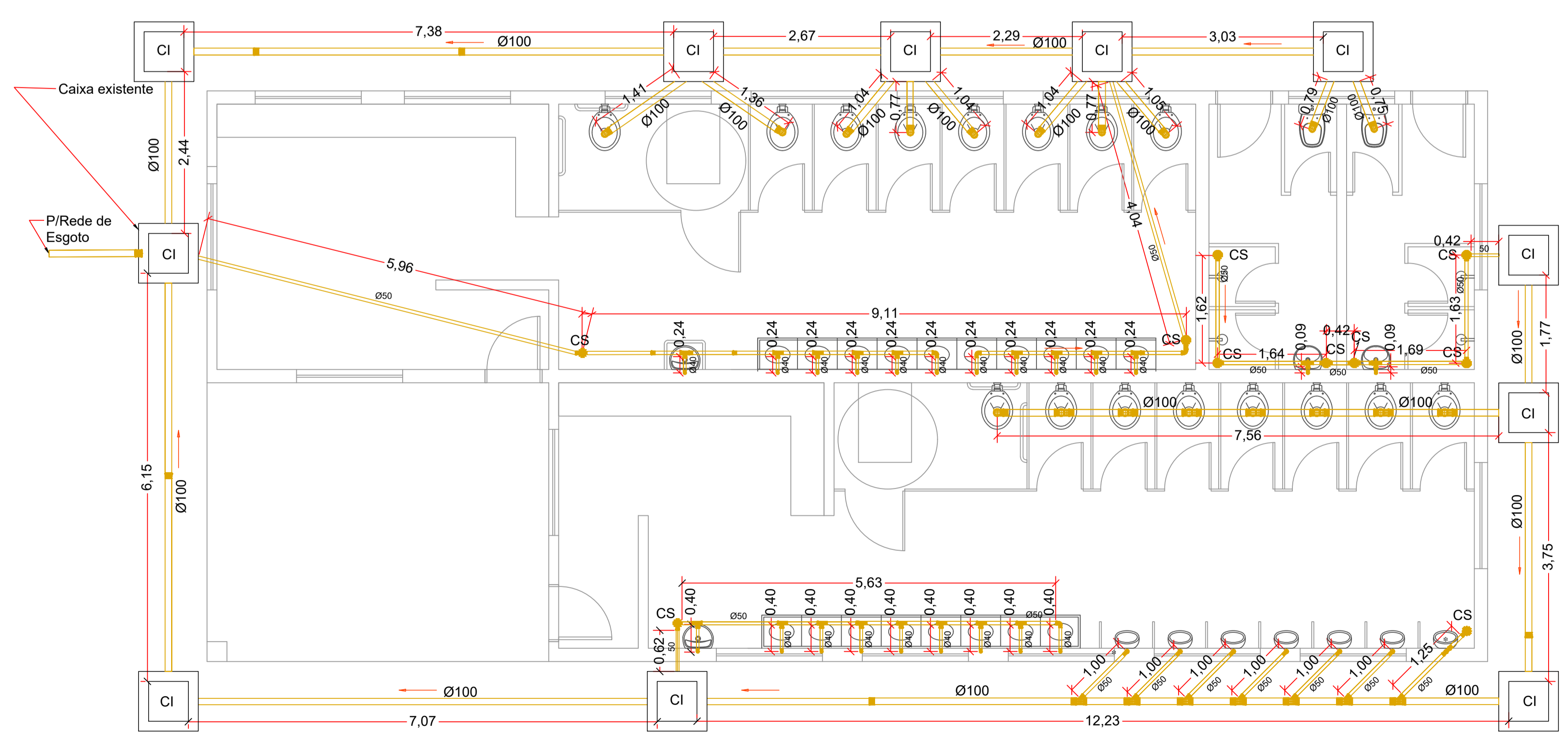
PLANTA REDE DE ESGOTO ESCALA 1:50
