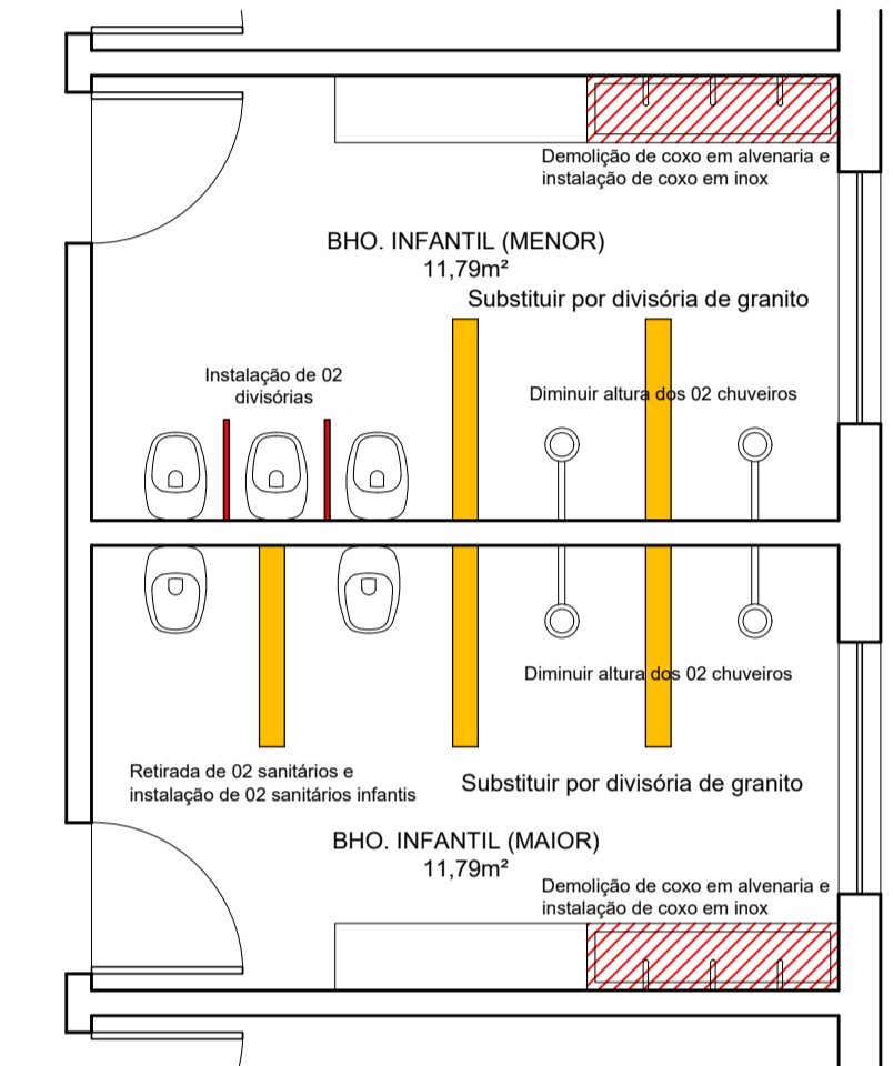
DETALHE SANITÁRIOS ESCALA 1/50
