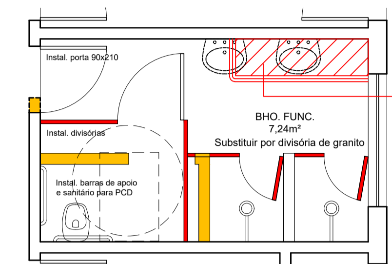
DETALHE BANHEIRO FUNCIONÁRIOS ESCALA 1/50
