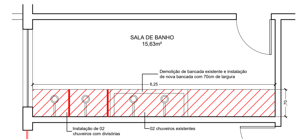
DETALHE SALA DE BANHO ESCALA 1/50
