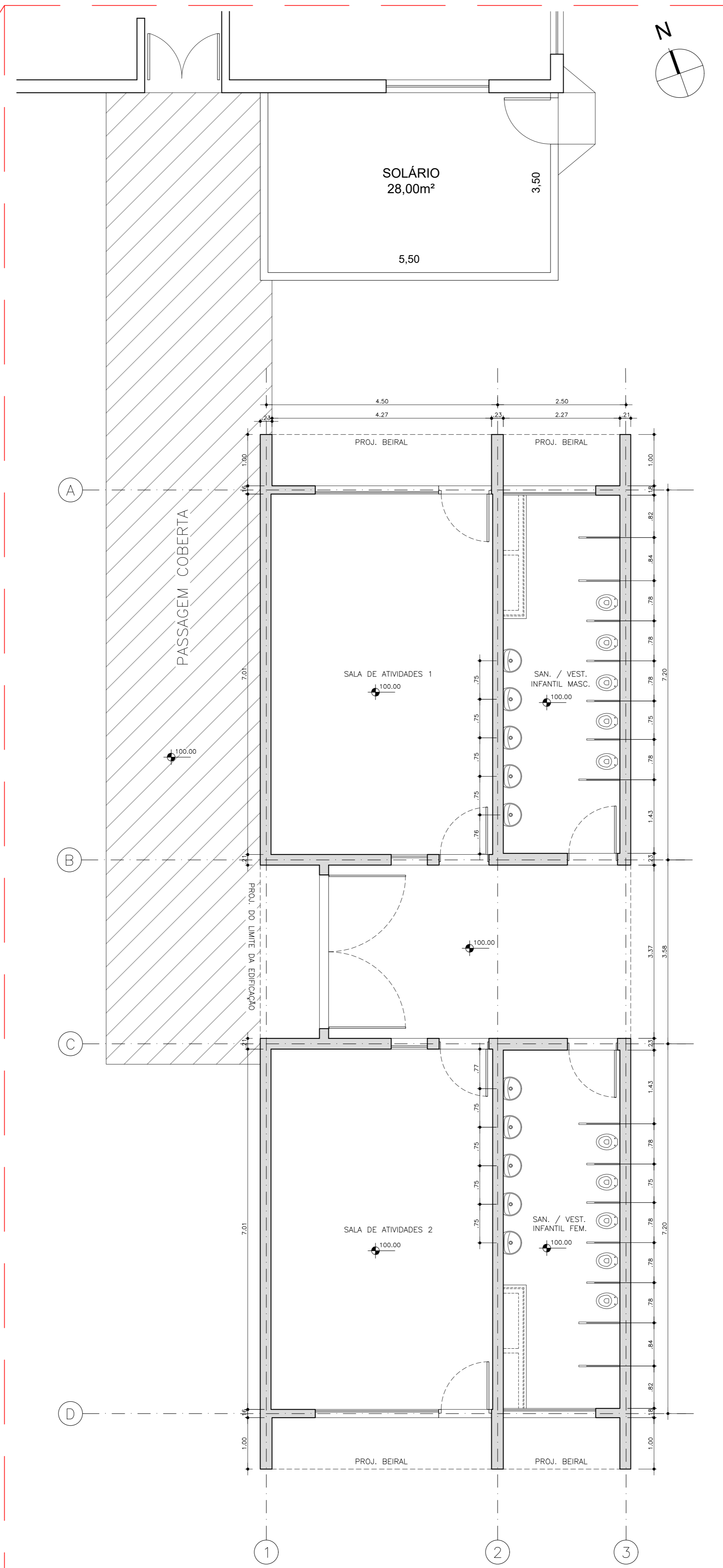
DET. PLANTA (ÁREA A CONSTRUIR) ESC 1:50
