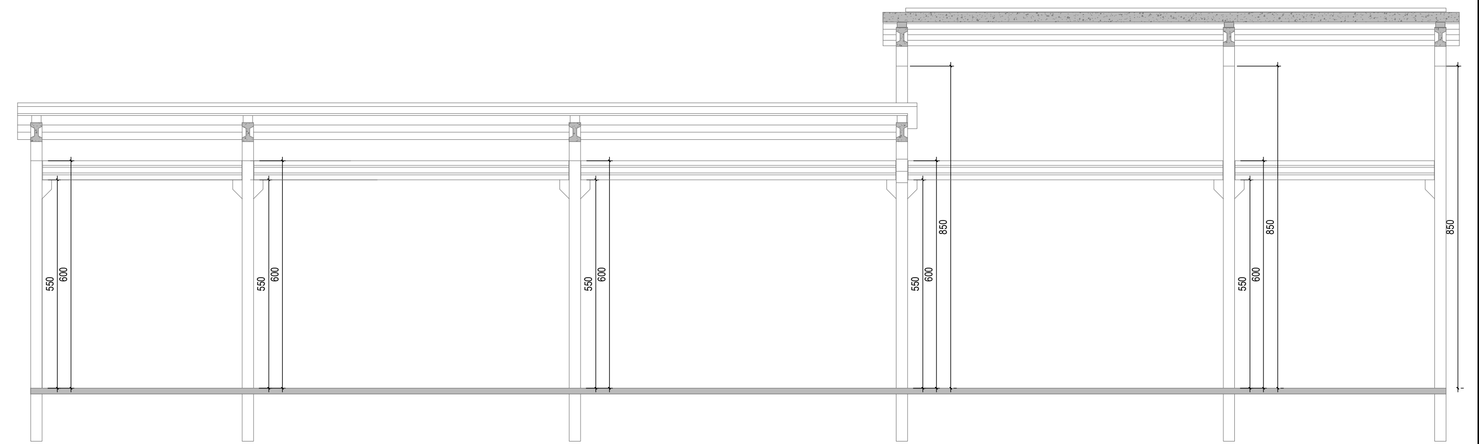
CORTE DD ESCALA 1:100
