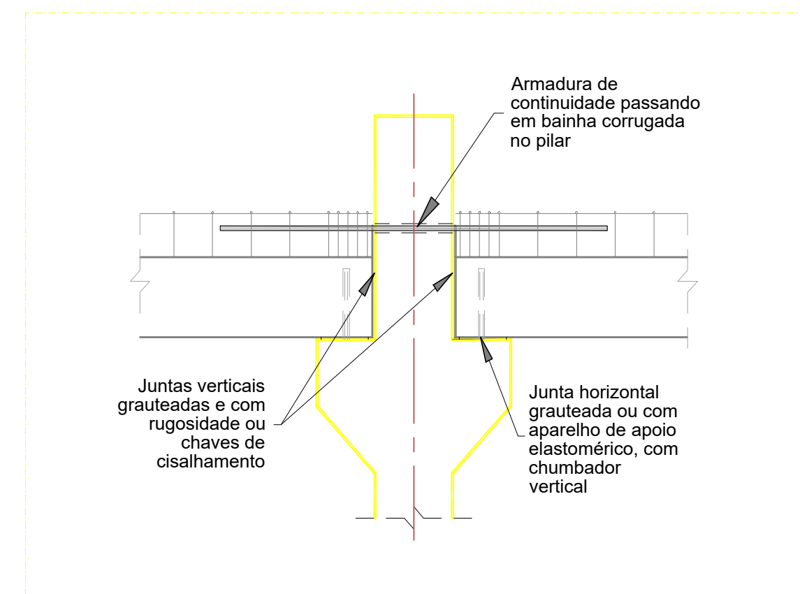
DETALHE 1 - LIGAÇÃO TÍPICA - VIGA-PILAR SEM ESCALA
