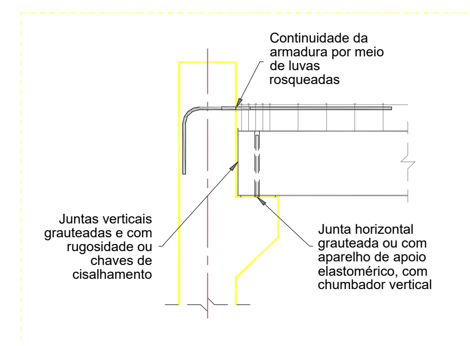
DETALHE 2 - LIGAÇÃO TÍPICA - VIGA-PILAR SEM ESCALA
