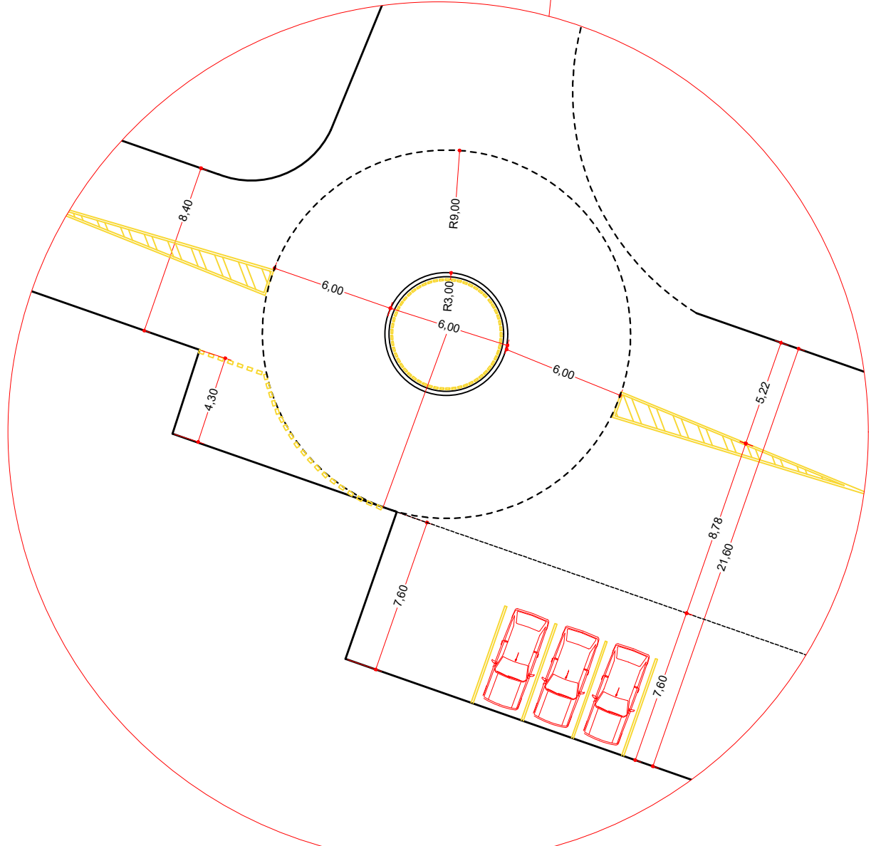
DETALHE MINIROTATÓRIA COM TACHÃO ESC 1/250
